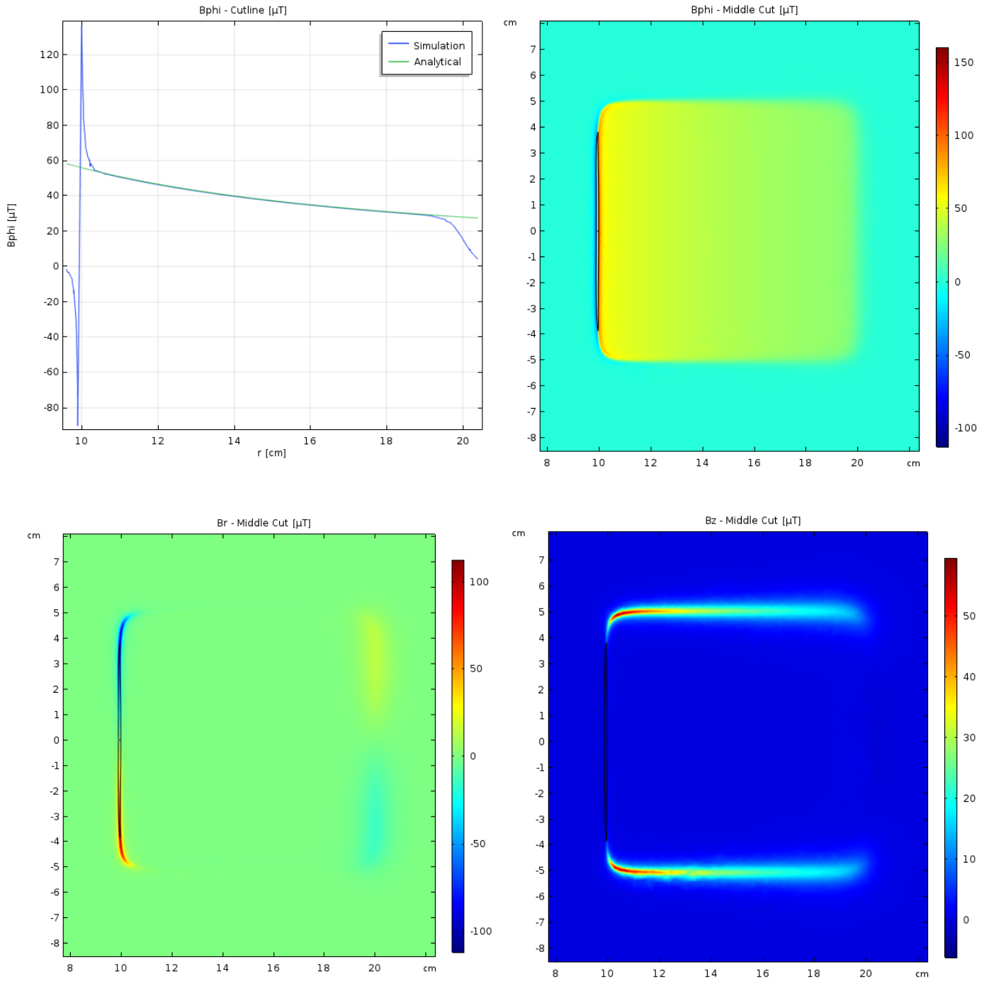
Kuva 1. Simulaatiotuloksia magneettivuon tiheydestä ( d_{in} = 20 cm, d_{out} = 40 cm, h = 10 cm, N = 100 , d_{wire} = 1 mm, I = 0,28 A).
