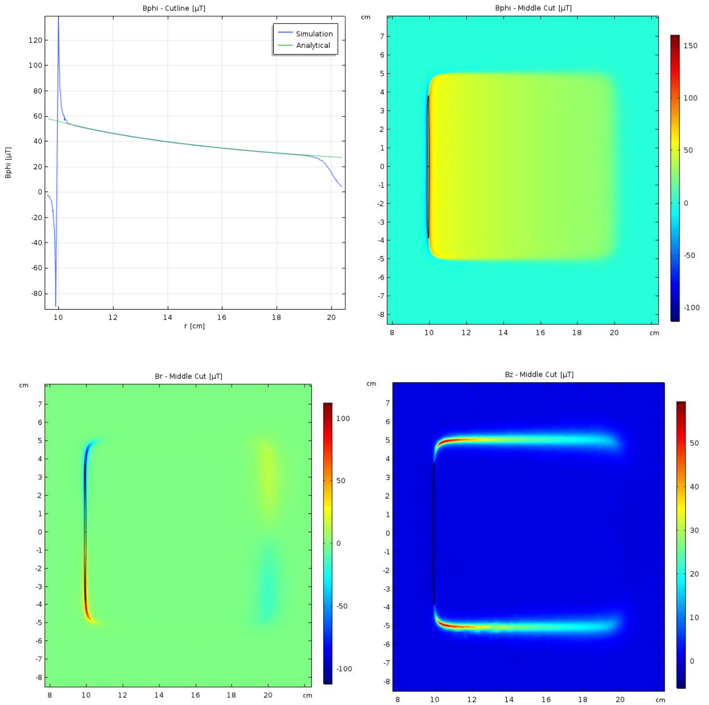
Figur 1. Simuleringsresultat för den magnetiska flödestätheten ( d_{in} = 20 cm, d_{out} = 40 cm, h = 10 cm, N = 100 , d_{wire} = 1 mm, I = 0,28 A).
